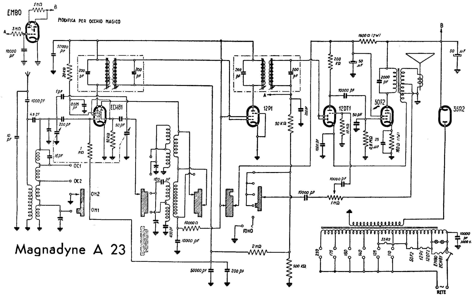
MAGNADYNE RADIO - Modd. A 23 e K 423. Apparecchio a gamma onde medie divisa, e gamma onde corte divisa. Media frequenza a 471 kc/s. Potenza d'uscita 2 watt.
